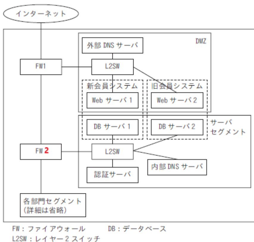
図1 K社のシステム構成の概要
